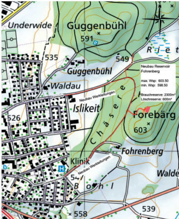
Situations- / Projektübersichtsplan Bauzone bis Reservoir
