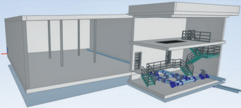
Visualisierung Schnitt Wasserkammer und Bedienhaus mit Installationen
