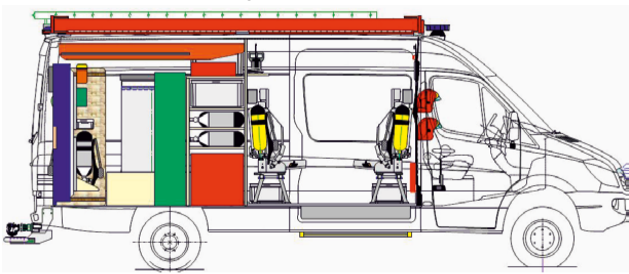
Atemschutzfahrzeug Feuerwehr Aadorf Seitenansicht rechts
